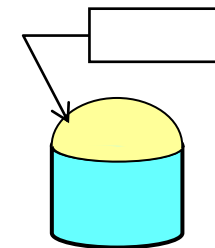
Sphère
