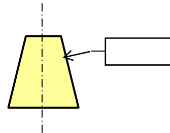
Cône
